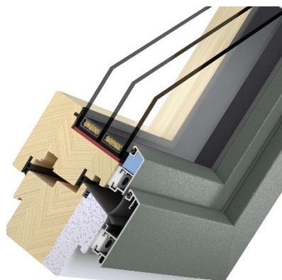
SOLID (Flächenversetzt)
