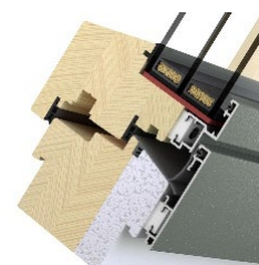
SLIM (Flächenbündig)
